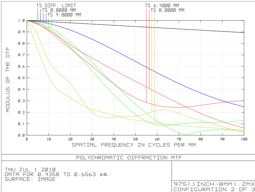
MTF (Object 1.0m)/ F1.4
